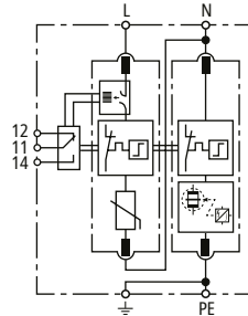
Prinzip Schaltbild DG M TT 2P ACI 385 FM
