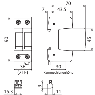
Maßbild DG M TT 2P ACI 385 FM
