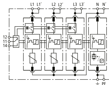
Prinzipschaltbild DG MD TT ACI 275 FM
