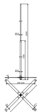
Maßbild FS 16 10 2000 MD AL V2A
