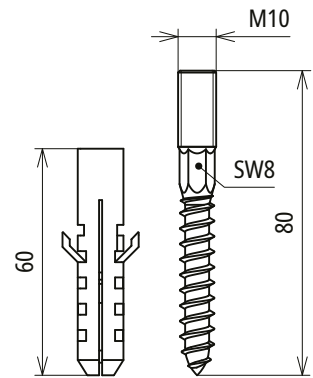
Maßbild BFS M10X20 PAS STTZN
