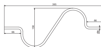
Maßbild DS 8 L395 AL
