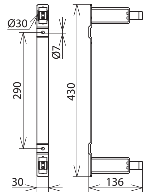
Maßbild HV P ST D30
