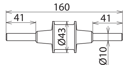
Maßbild TFS
