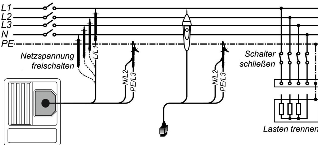
Abbildung 5.6: Anschluss der 3-Leiter-Prüfleitung und der optionalen Commander-Prüfspitze (044155)
