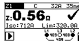
Abbildung 5.29: Beispiel Leitungsimpedanzmessung
