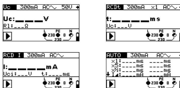
Abbildung 5.16: FI/RCD-Prüfungen
