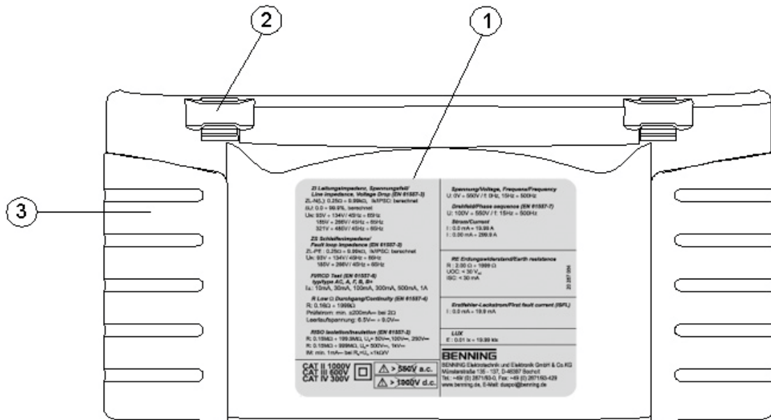
Abbildung 3.5: Bodenansicht
