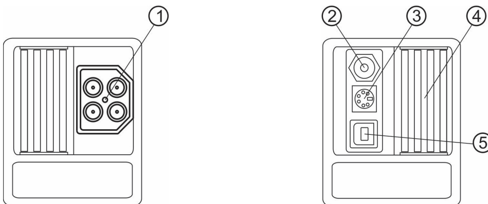
Abbildung 3.2: Anschlussfeld
