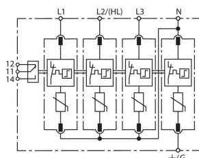
Prinzipschaltbild DG MU 3PH 240 4W+G R
