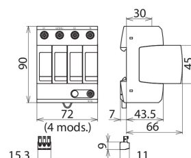
Maßbild DG MU 3PH 240 4W+G R
