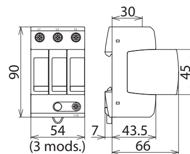
Maßbild DG MU 3PD 480 3W+G
