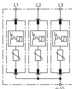
Prinzipschaltbild DG MU 3PD 480 3W+G
