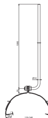
Maßbild FS 10 1000 FG AL V2A
