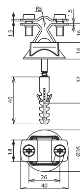
Maßbild LH ZS 8.10 FL20 KS KD8X40 CU
