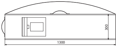
Maßbild KLT 133 34 10
