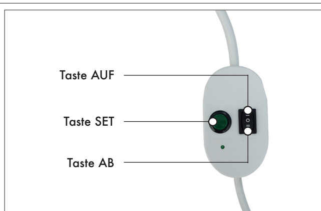
Abb.5: Justierschalter (Art.-Nr. 125400)
