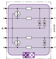
Prinzipschaltbild BXT ML4 BE BD 24
