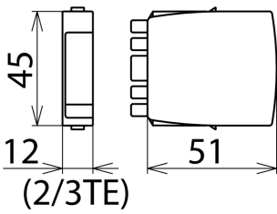
Maßbild BXT ML4 BE BD 24
