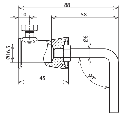
Maßbild BA90 RD8 BB16 V2A ZG
