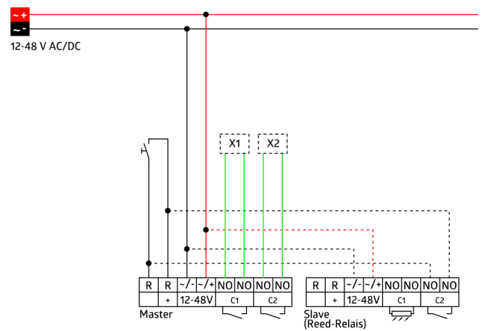
Schaltbild 92154
