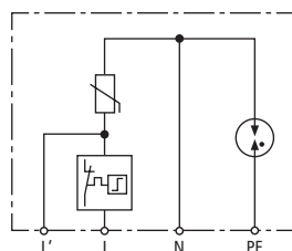
Prinzipschaltbild DCOR L 2P SN1860
