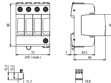
Maßbild DG MD TT 275 FM
