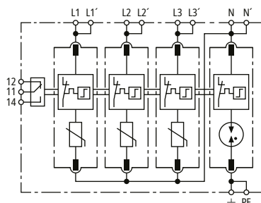
Prinzipschaltbild DG MD TT 275 FM
