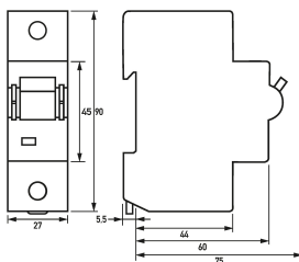
Maßzeichnung Gruppenansicht
