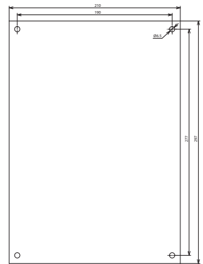
Maßbild HWS 297X210 AGU3MV DE EN AL
