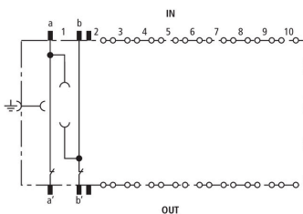
Prinzip Schaltbild BM 10 DRL
