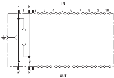
Prinzipschaltbild BM 10 DRL
