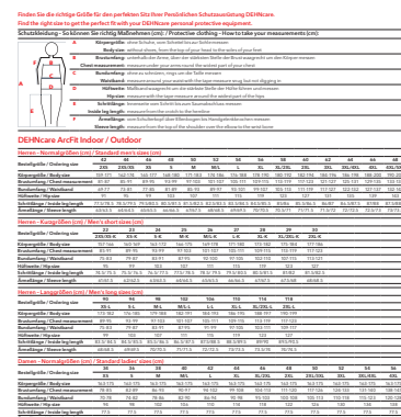
Maßbild APJ ID F 34
