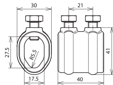
Maßbild TM 7.10 16 RG
