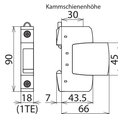
Maßbild DG S 150
