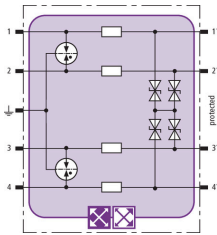
Prinzipschaltbild BXT ML4 BC 5
