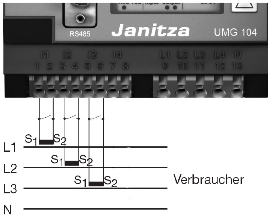
Abb.: Beispiel - Anschlusschema Strommessung UMG 104 Utility Meter mit Messwandlern
