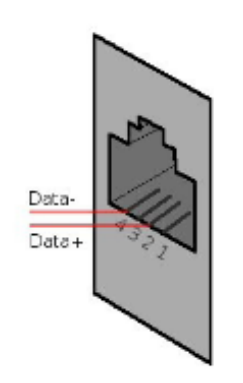
Abb.: Pinbelegung RJ14 Buchse
