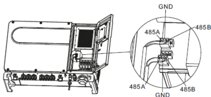
Abb.: Klemmleistenblock im Wechselrichter
