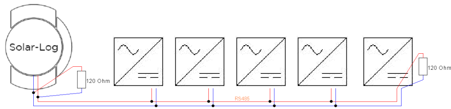
Abb.: Beispiel 1 einer Bus-Topologie
