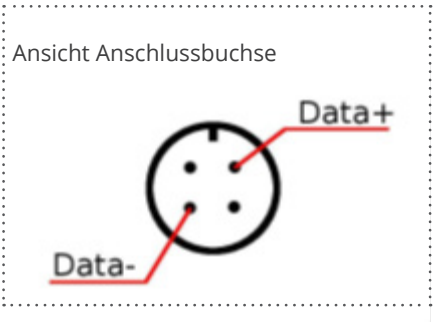
Abb.: Rund-Buchse Fronius RL
