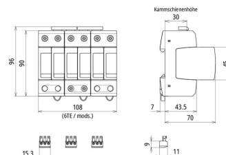
Maßbild DG M DC ACI 1250 FM
