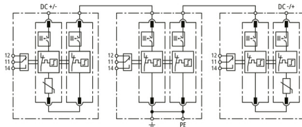
Prinzipschaltbild DG M DC ACI 1250 FM
