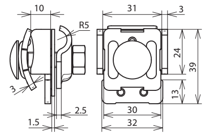
Maßbild ZMFK KB 6.10 KBF0.7 8 CU STTZN
