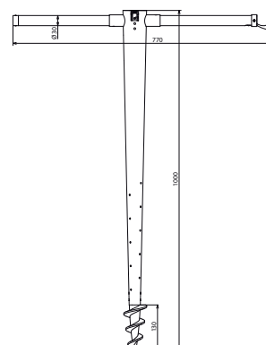
Maßbild ERO BSP ASSM10 1000 STTZN
