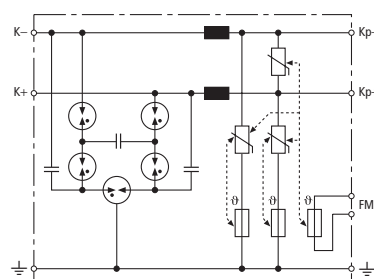
Prinzipschaltbild BVT KKS ALD 75
