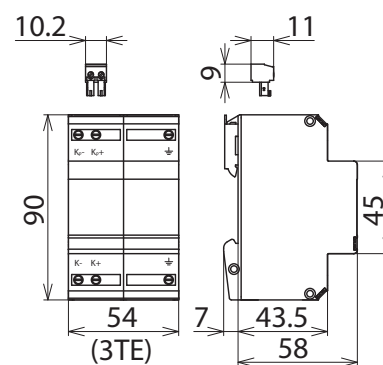
Maßbild BVT KKS ALD 75
