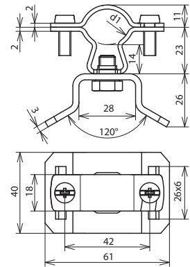
Maßbild LH ZS 20 23 SBH 25X0.3 V2A
