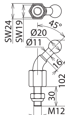
Maßbild KFP 20 W45M12 SN7024
