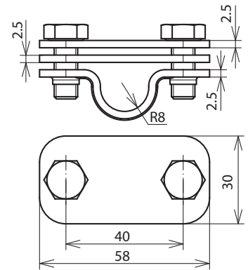
Maßbild UTK 16 FL30 ZP V2A
