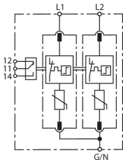
Prinzip Schaltbild DG MU SP 240 3W+G R
