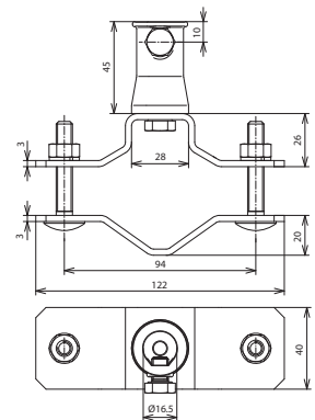
Maßbild RS D40.60 BB16 V2A ZG
