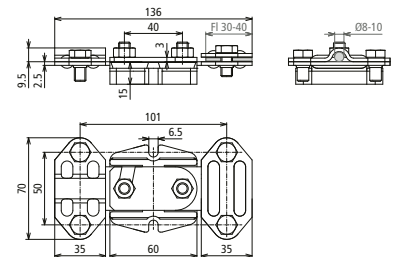
Maßbild FTS 8.10 FL30.40 IS STTZN
