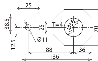
Maßbild AB EXFS IF3 G 36
