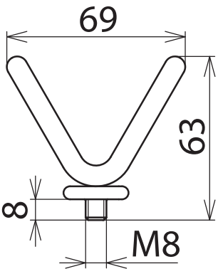
Maßbild EL M8 G PHE
