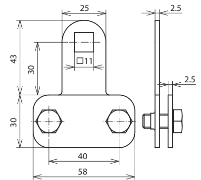
Maßbild KS B11.11 FL30X4 V2A
