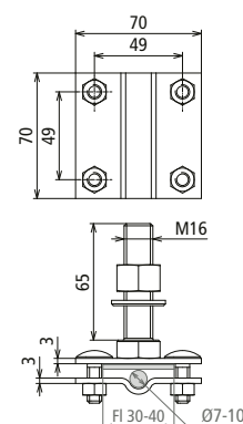
Maßbild AK 7.10 FL40 GBM16X65 V4A
