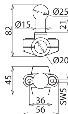
Maßbild KFP 25 RL 20
