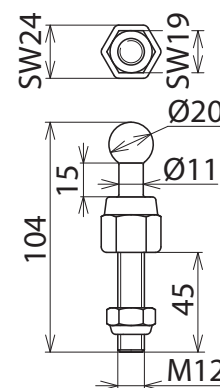
Maßbild KFP 20 M12 45 SN7078
