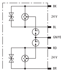
Prinzipschaltbild DPI CD EXI+D 2X24 N
