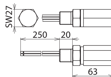
Maßbild DPI CD EXI+D 2X24 N
