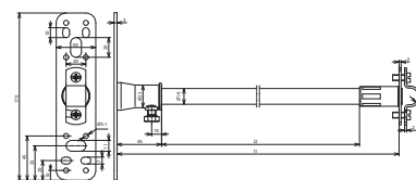
Maßbild DIDH 16 690 BP V2A GFK
