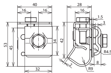
Maßbild ZMDRK DUL 8.10 W16.22 CU STTZN
