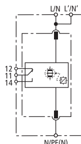
Prinzipschaltbild DB M 1 150 FM
