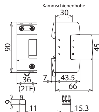
Maßbild DB M 1 150 FM
