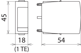
Maßbild DG MOD ACI 385
