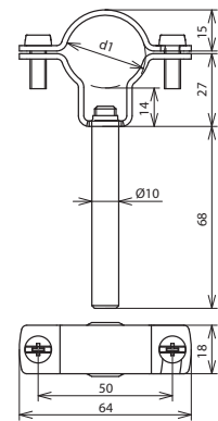
Maßbild LH ZS 27 DS10 L75 V2A
